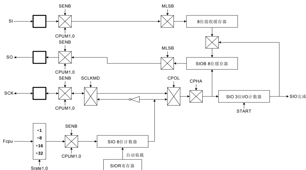
SIO 接口示意图
